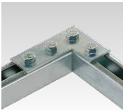
Placa angular
